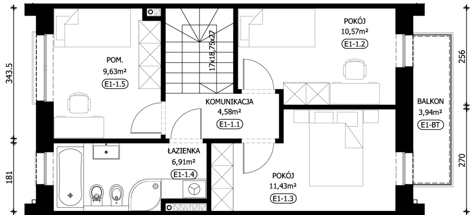
RZUT PIĘTRA
