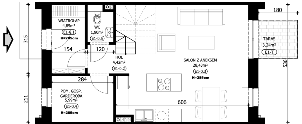
RZUT PARTERU
