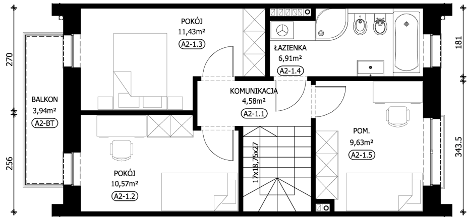
RZUT PIĘTRA
